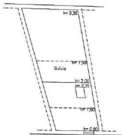
PIANO SECONDO sottotetto
