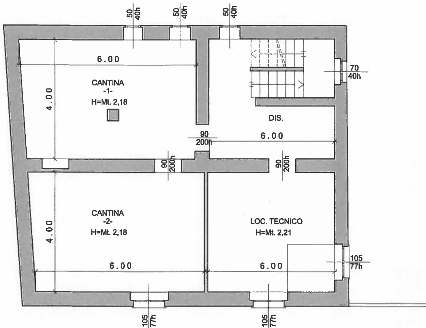
PIANO PRIMO SOTTOSTRADA - stato di progetto-
