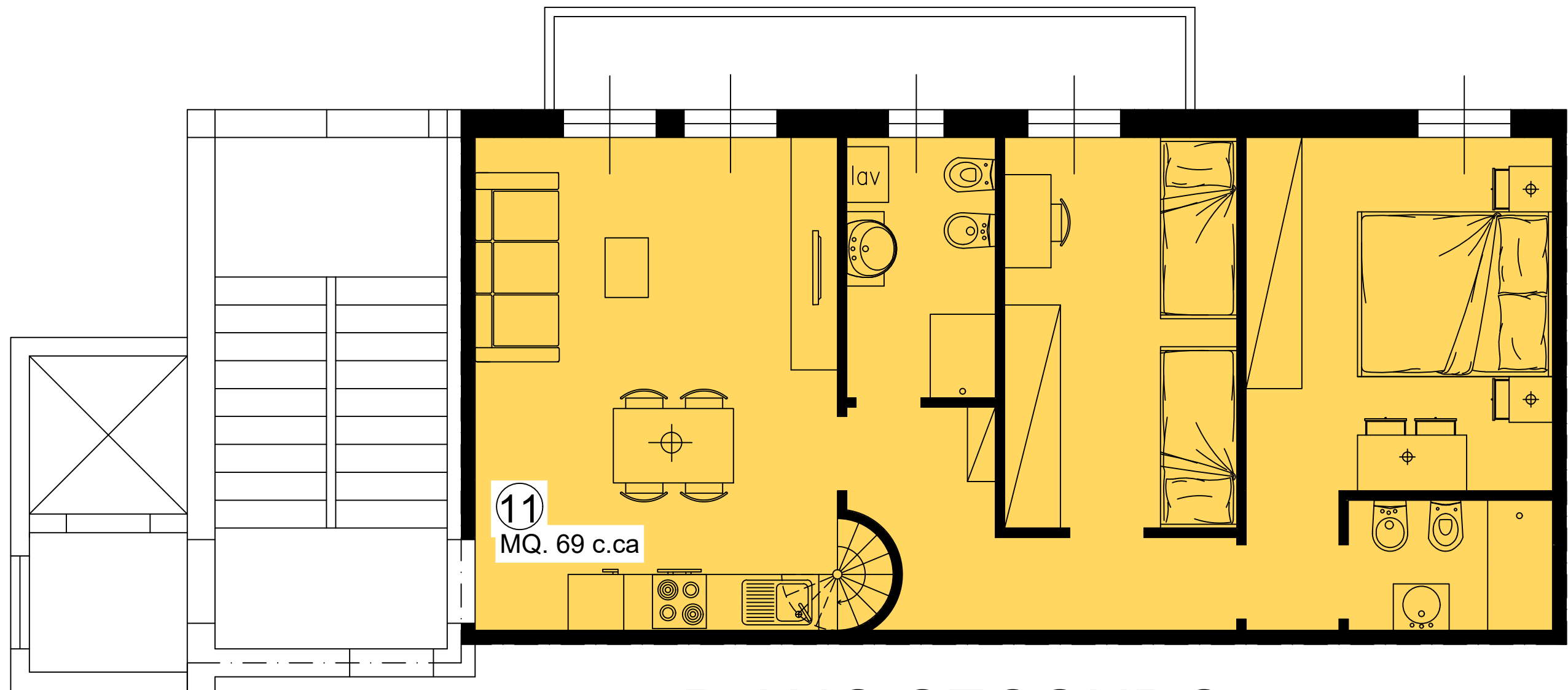
PIANO SECONDO
