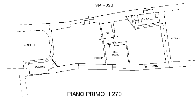
PIANO PRIMO H 270
