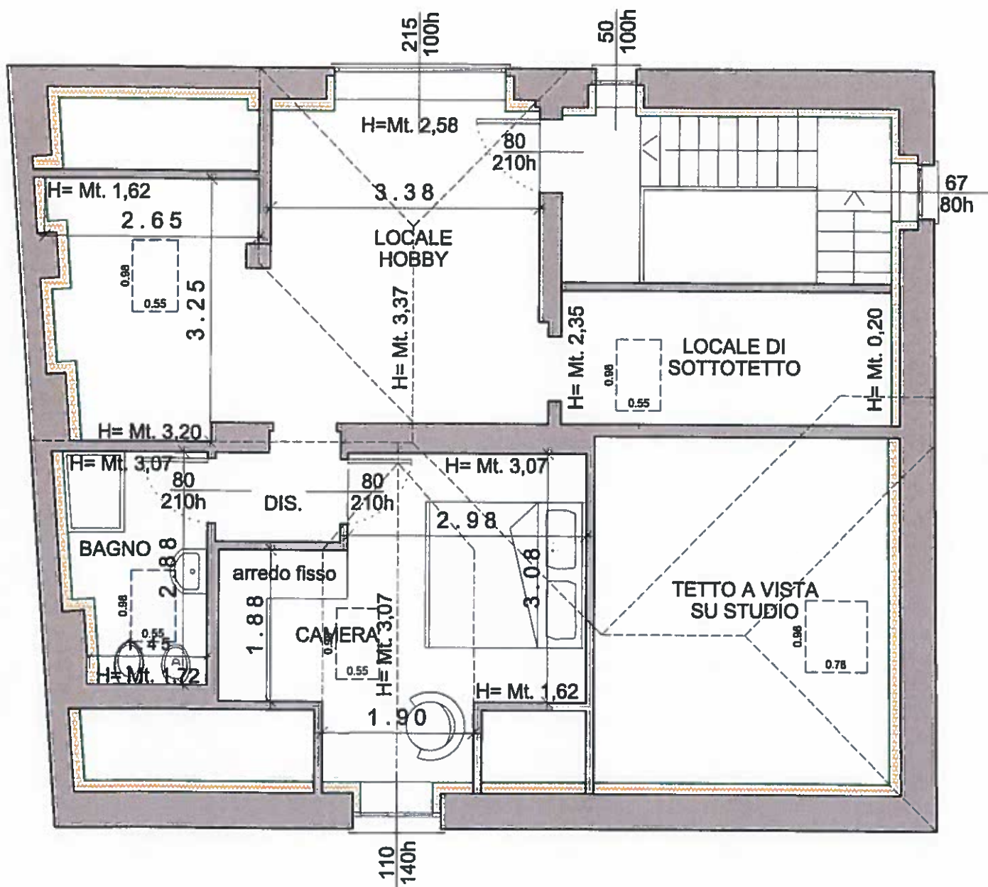
PIANO SOTTOTETTO - progetto -
