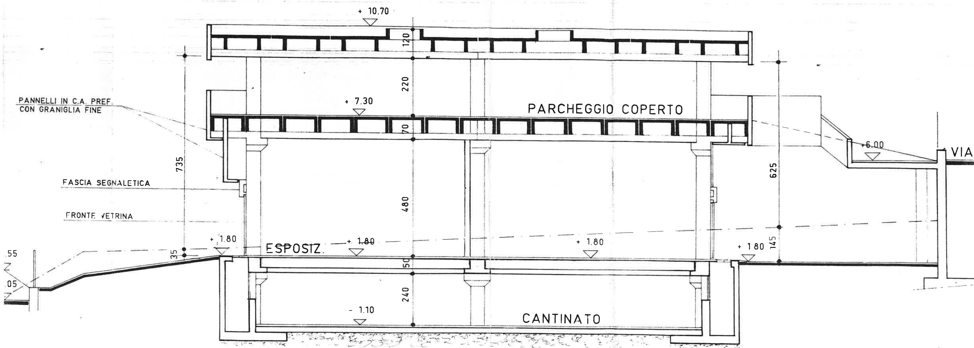
SEZIONE GG'
