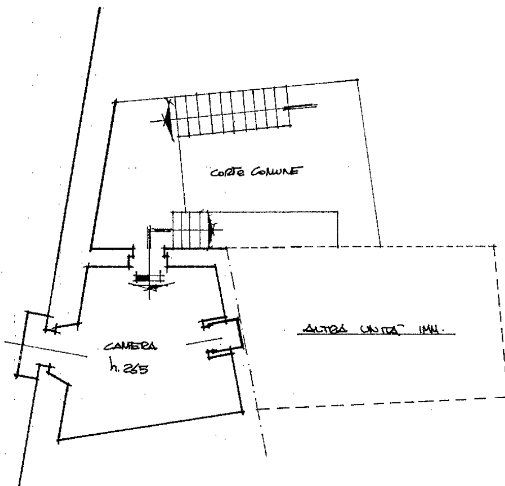
PIANO PRIMO
