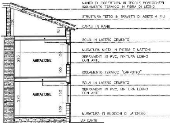
SEZIONE -A- STATO DI PROGETTO
