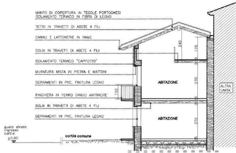
SEZIONE -B- STATO DI PROGETTO
