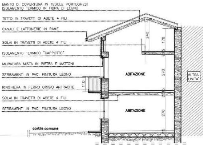
SEZIONE -A- STATO DI PROGETTO
