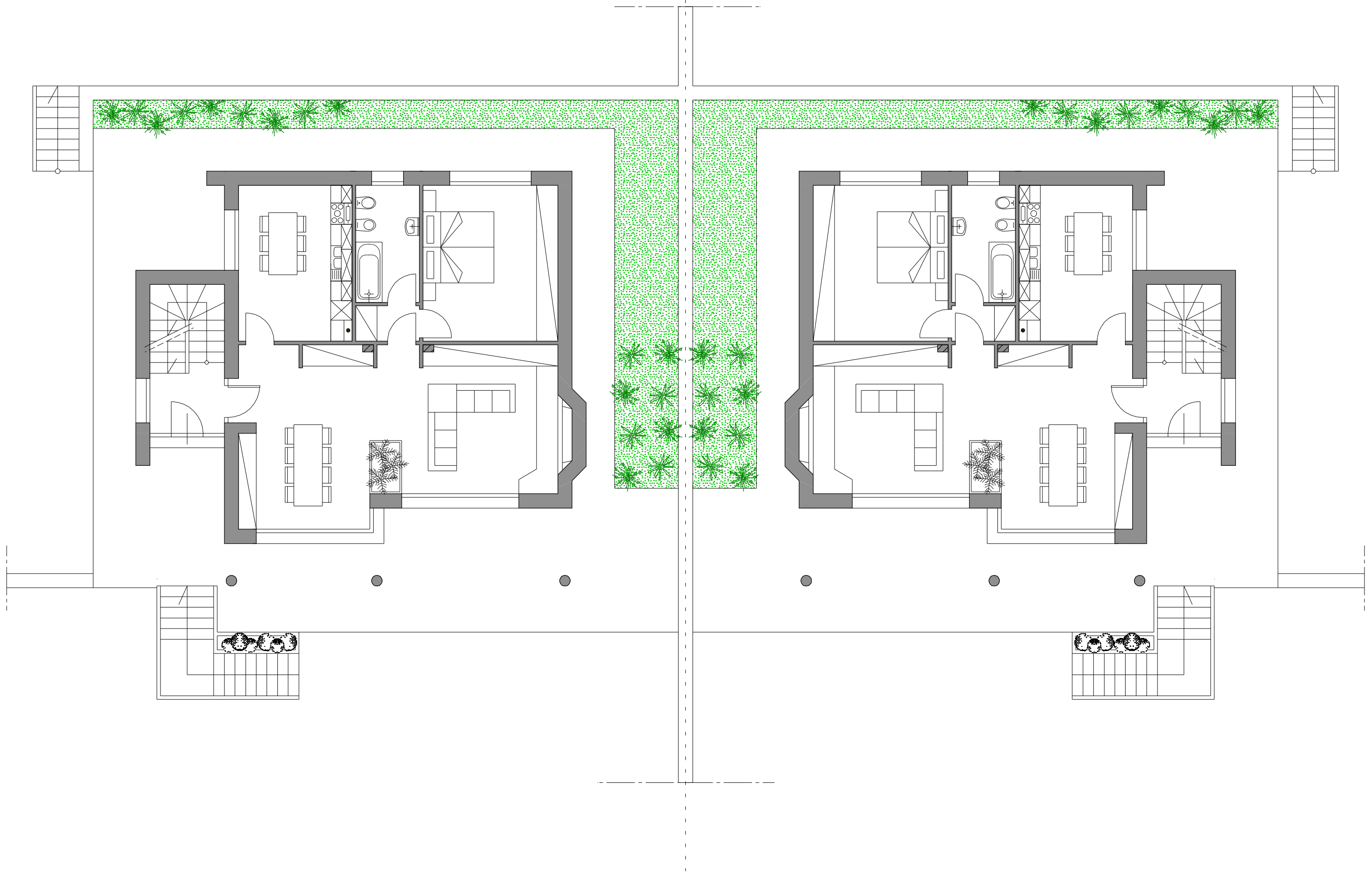
PIANTA PIANO TERRA SC: 1:100
