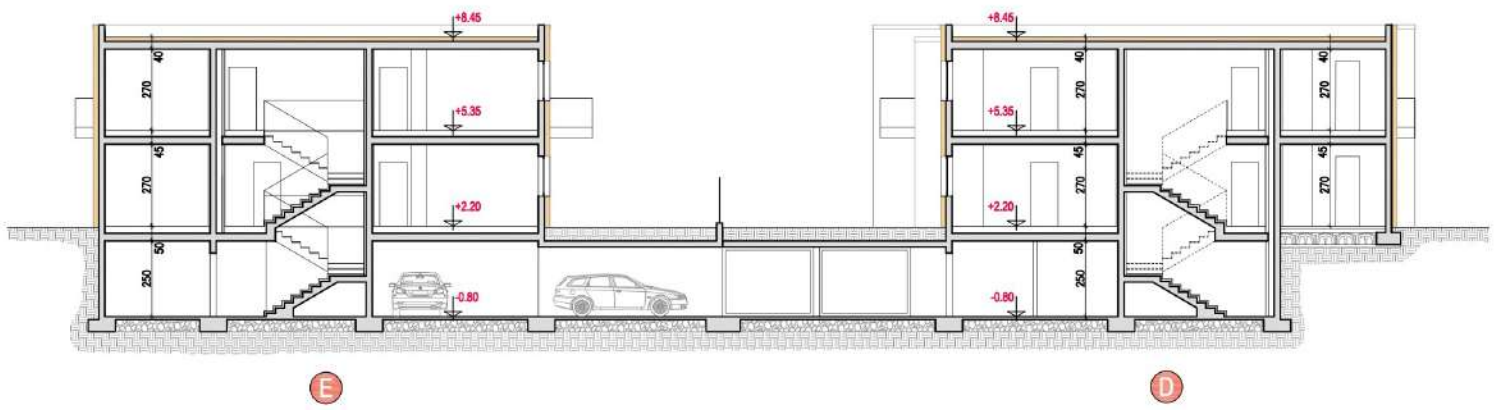
SEZIONE A-A
